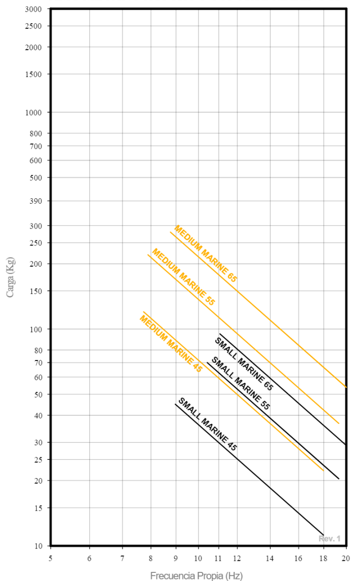
FRECUENCIA PROPIA AMC MECANOCAUCHO® SOPORTE MARINO X
