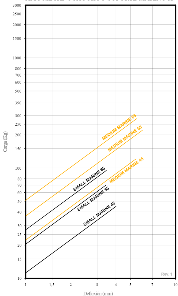
CURVAS DE CARGA FLECHA AMC MECANOCAUCHO® SOPORTE MARINO X
