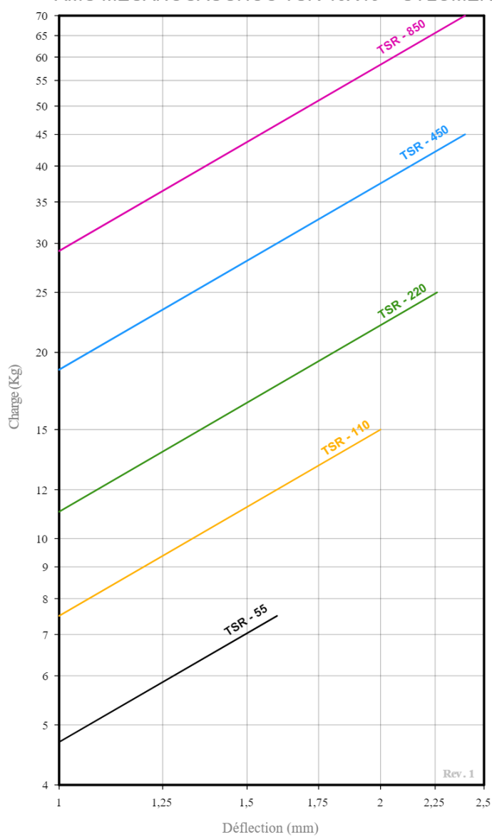
COURBE DE CHARGE FLÈCHE AMC MECANOCAUCHO® TSR 40X40 + SYLOMER
