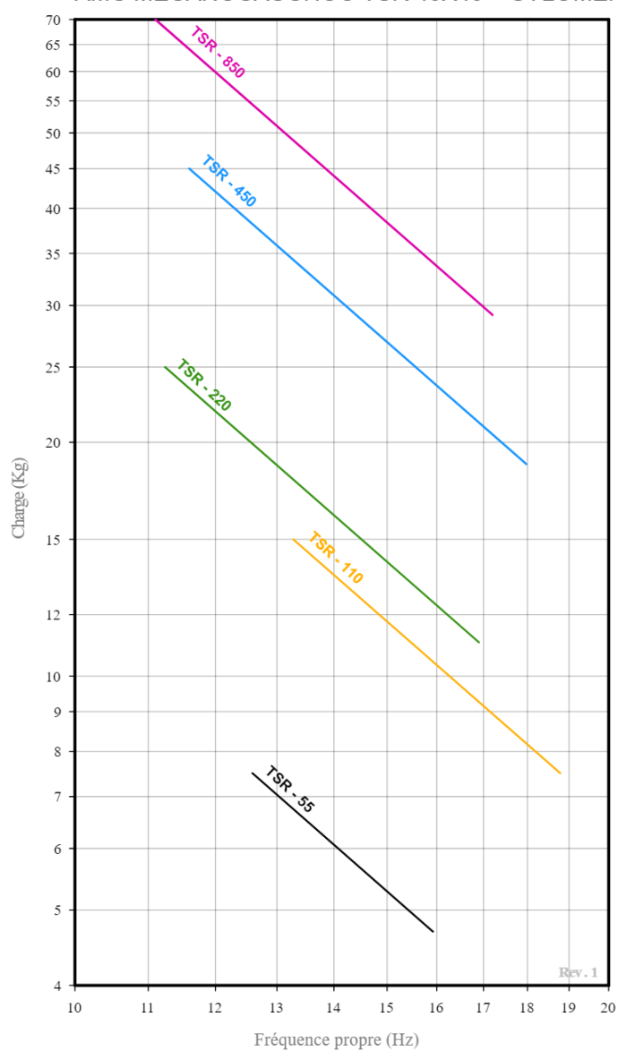
COURBE DE FRÉQUENCE PROPRE AMC MECANOCAUCHO® TSR 40X40 + SYLOMER
