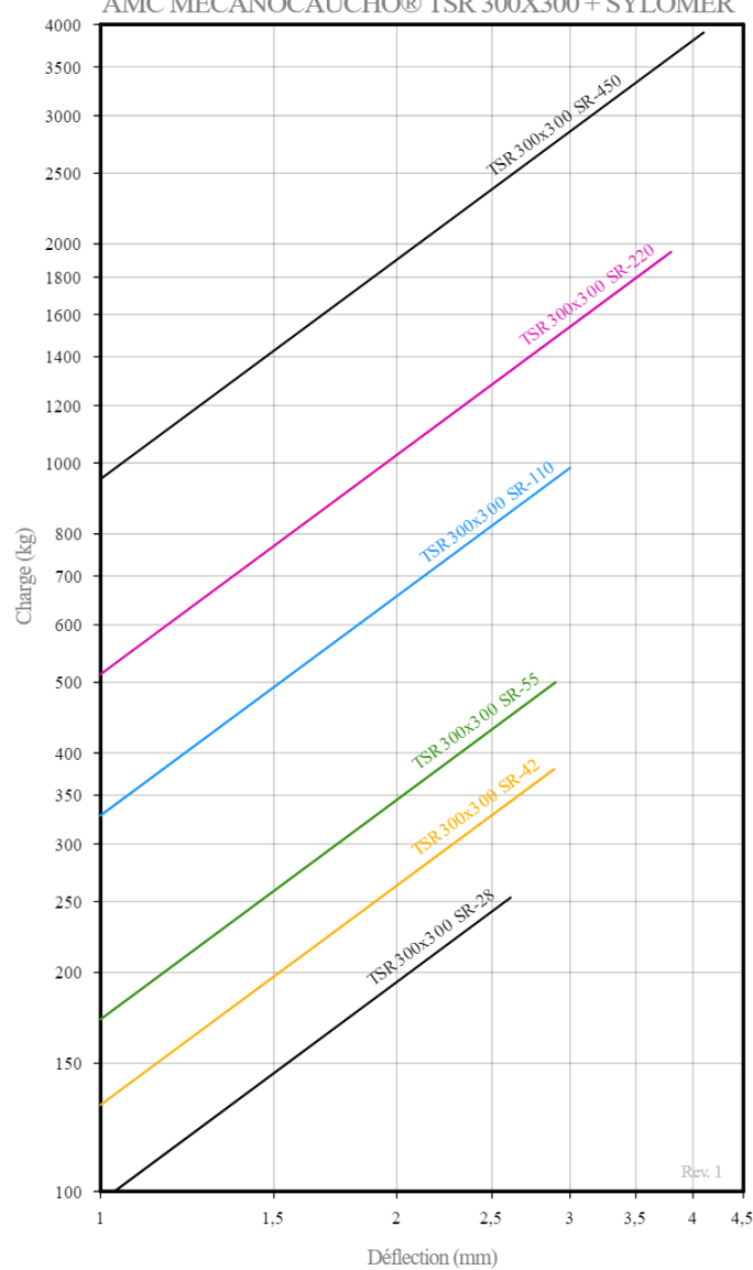
COURBE DE CHARGE FLÈCHE AMC MECANOCAUCHO® TSR 300X300 + SYLOMER
