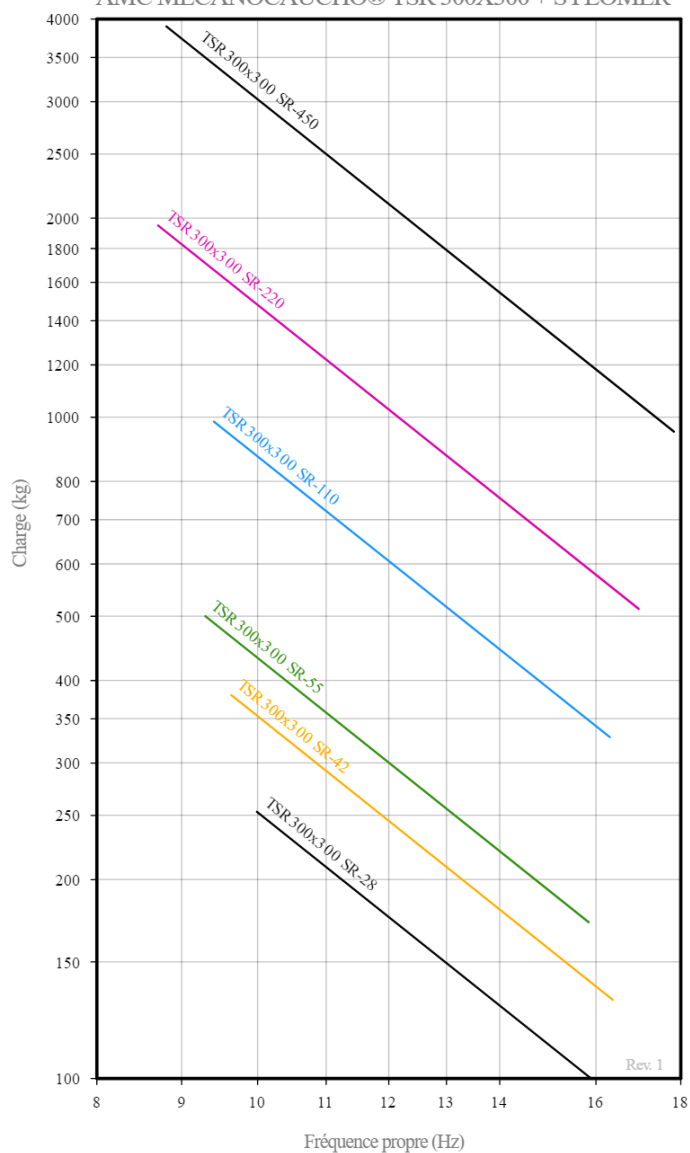
COURBE DE FRÉQUENCE PROPRE AMC MECANOCAUCHO® TSR 300X300 + SYLOMER
