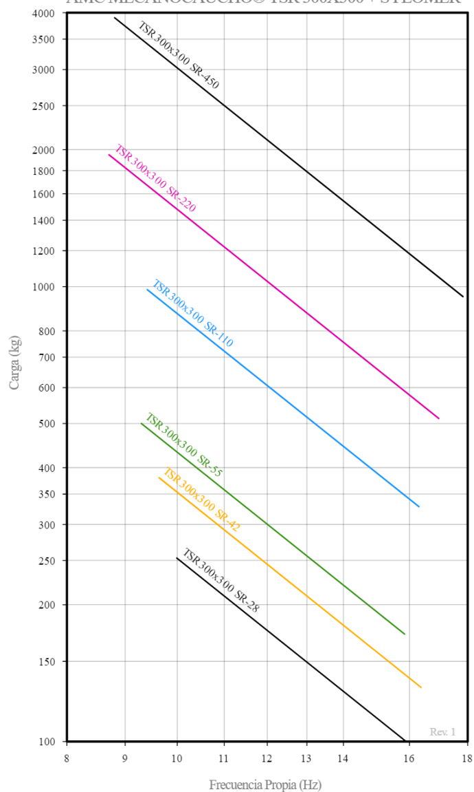
FRECUENCIA PROPIA AMC MECANOCAUCHO® TSR 300X300 + SYLOMER
