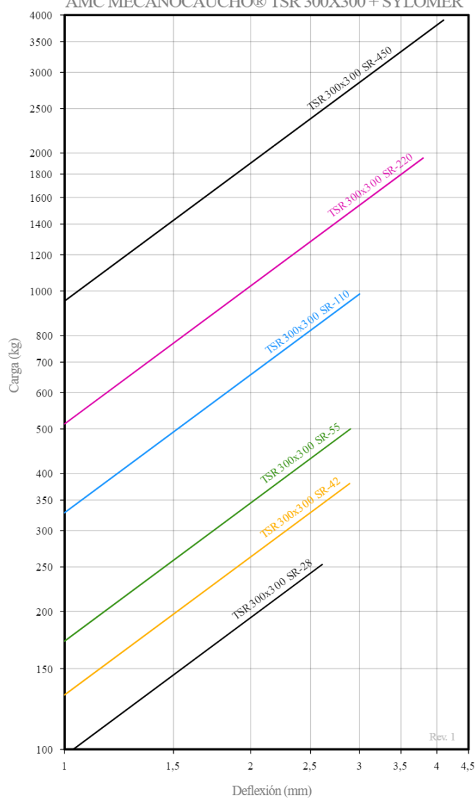
CURVAS DE CARGA FLECHA AMC MECANOCAUCHO® TSR 300X300 + SYLOMER
