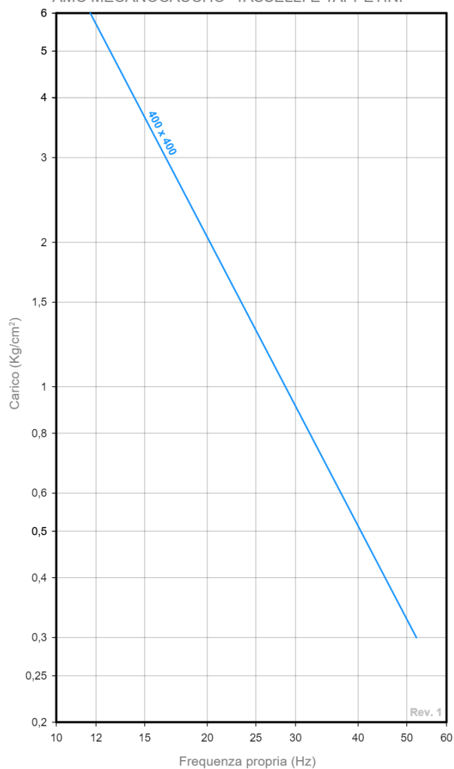
FREQUENZA PROPRIA AMC MECANOCAUCHO® TASSELLI E TAPPETINI
