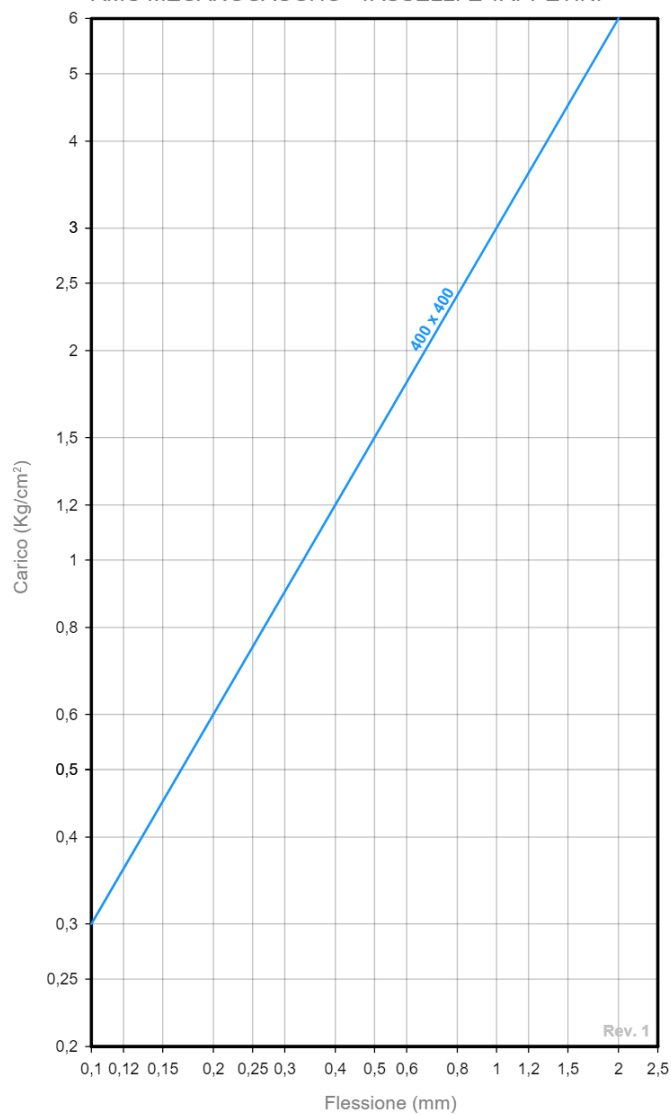
CURVE CARICO FLESSIONE AMC MECANOCAUCHO® TASSELLI E TAPPETINI
