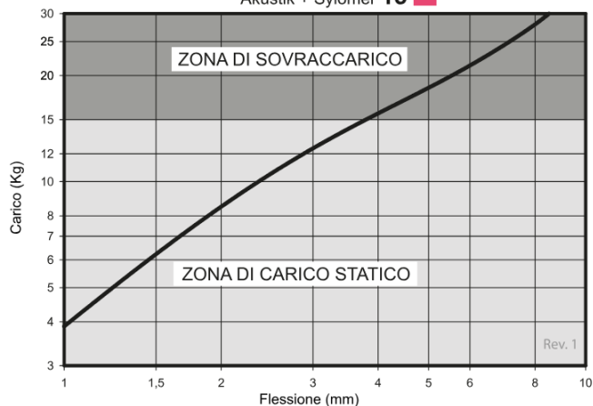
CURVE CARICO FLESSIONE
