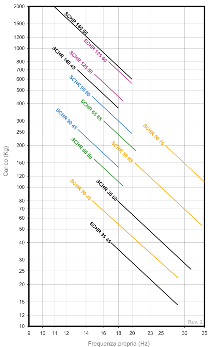
FREQUENZA PROPRIA AMC MECANOCAUCHO® SCHR
