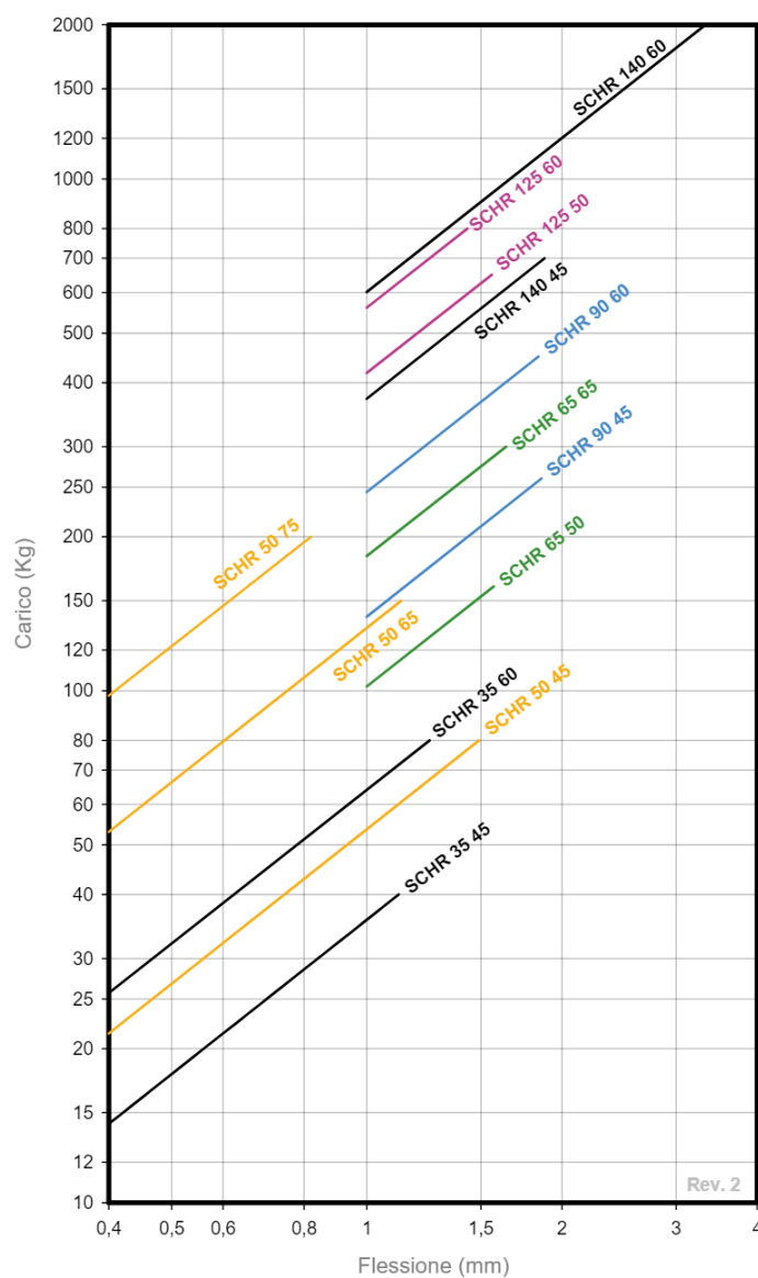
CURVE CARICO FLESSIONE AMC MECANOCAUCHO® SCHR
