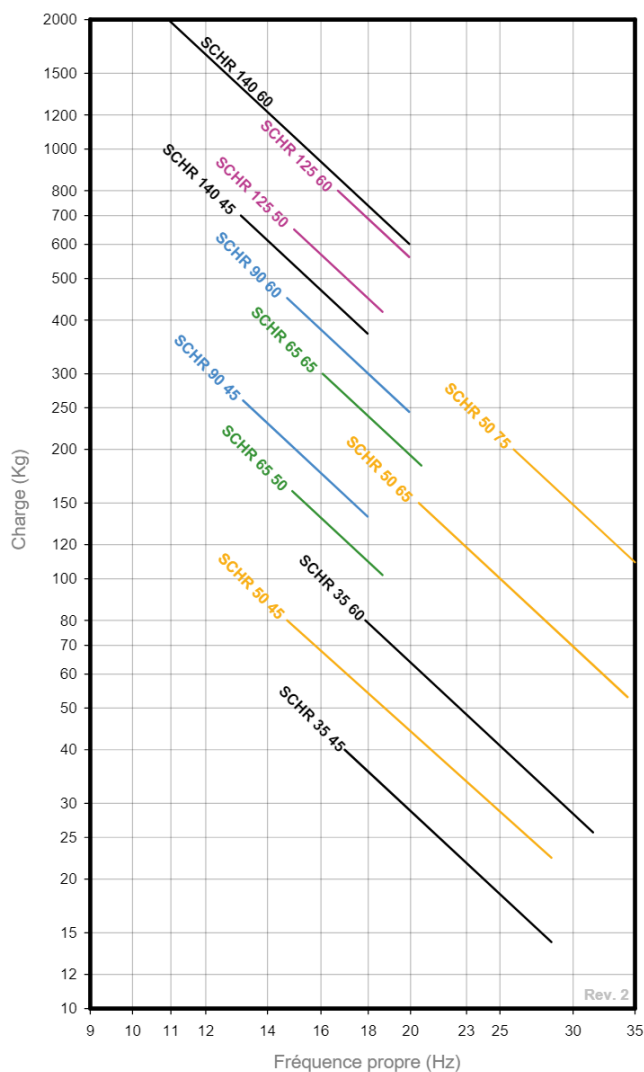
COURBE DE FRÉQUENCE PROPRE AMC MECANOCAUCHO® SCHR
