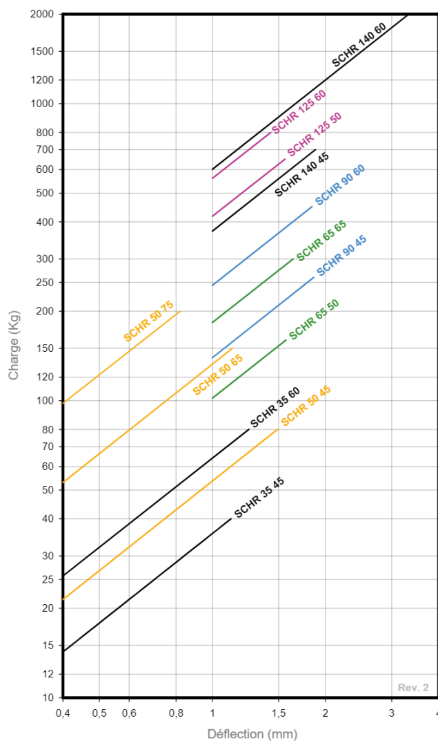
COURBE DE CHARGE FLÈCHE AMC MECANOCAUCHO® SCHR
