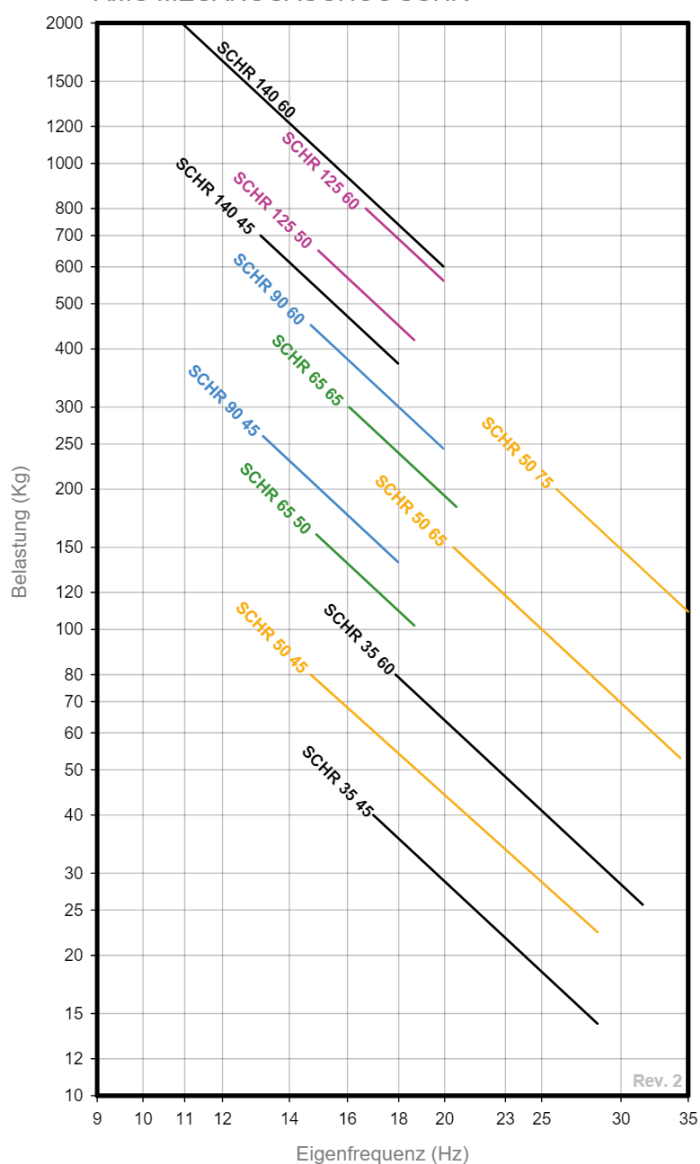
EIGENFREQUENZ AMC MECANOCAUCHO® SCHR
