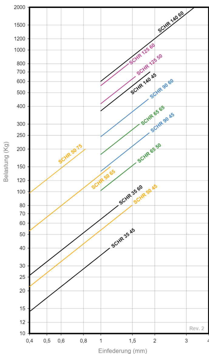
FEDERKENNLINIE AMC MECANOCAUCHO® SCHR
