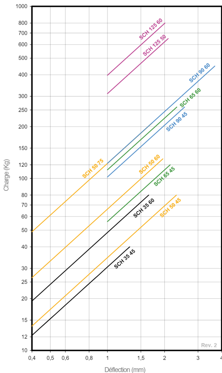
COURBE DE CHARGE FLÈCHE AMC MECANOCAUCHO® SCH
