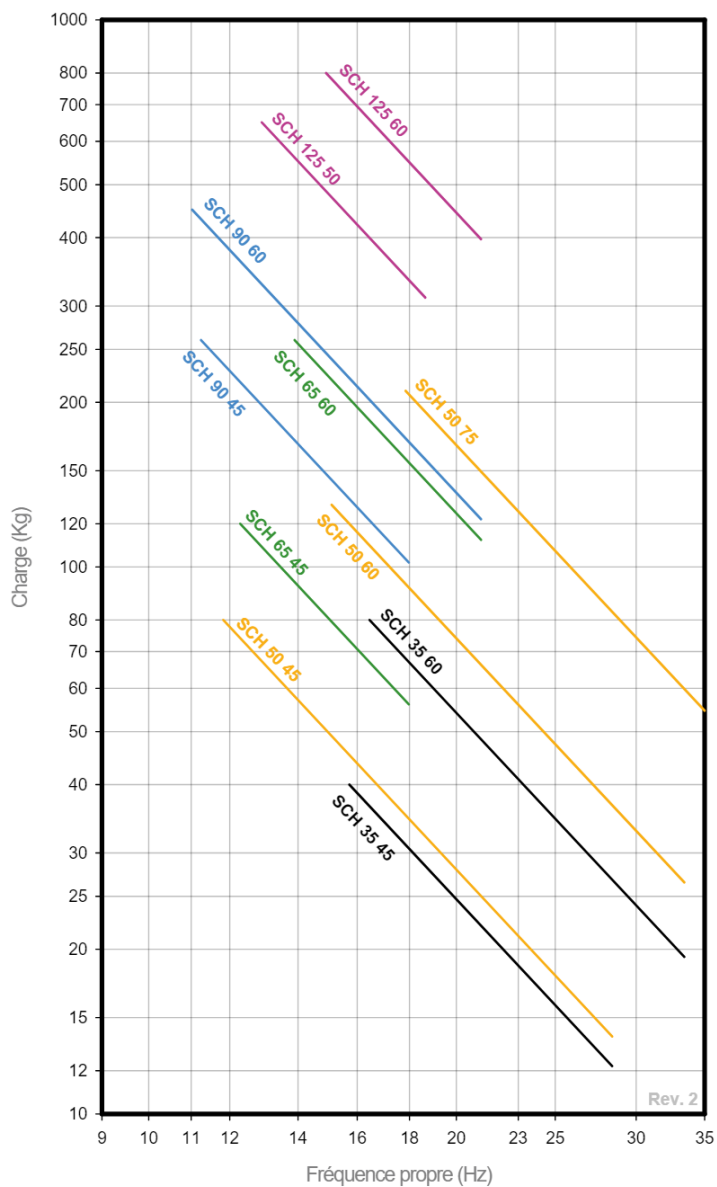
COURBE DE FRÉQUENCE PROPRE AMC MECANOCAUCHO® SCH
