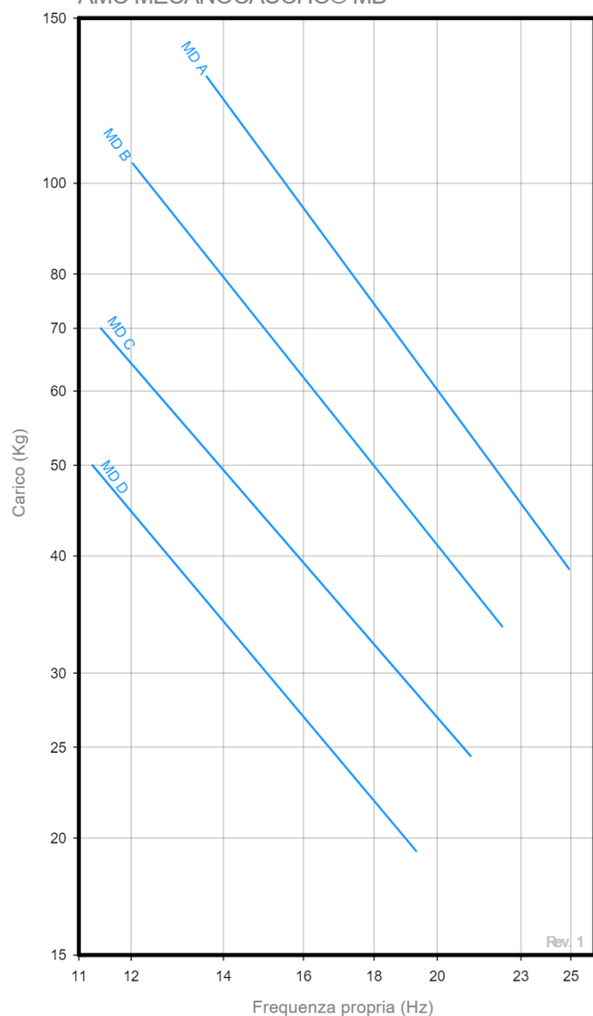
FREQUENZA PROPRIA AMC MECANOCAUCHO® MD
