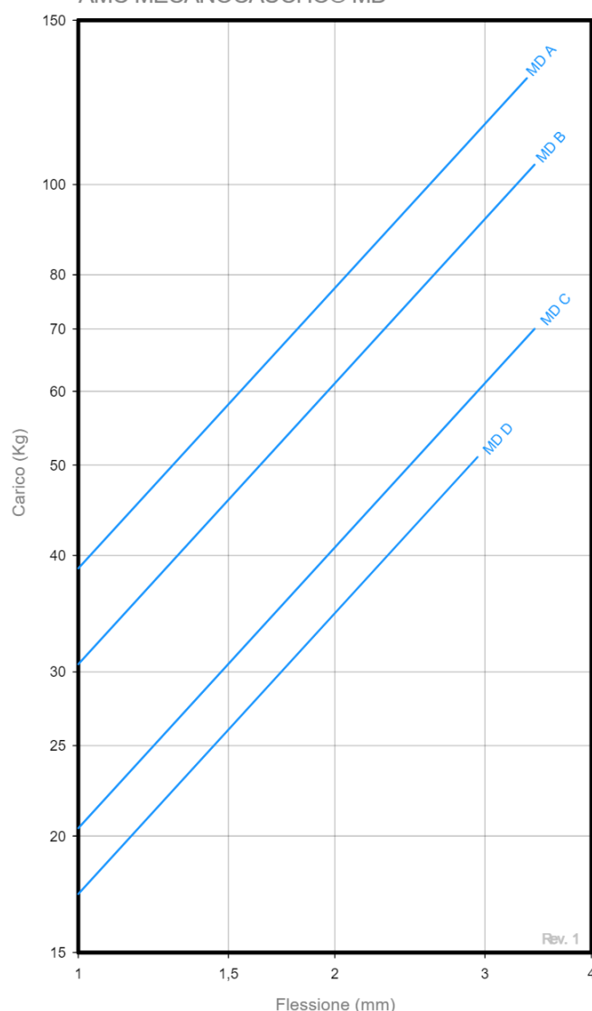
CURVE CARICO FLESSIONE AMC MECANOCAUCHO® MD
