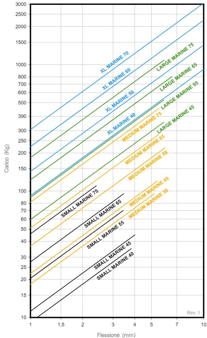
CURVE CARICO FLESSIONE AMC MECANOCAUCHO® SUPPORTI MARINI
