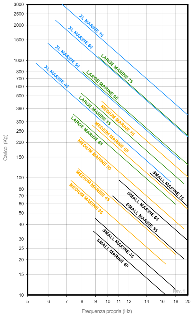
FREQUENZA PROPRIA AMC MECANOCAUCHO® SUPPORTI MARINI
