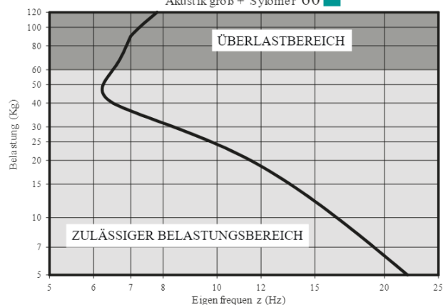
EIGENFREQUENZKURVE
