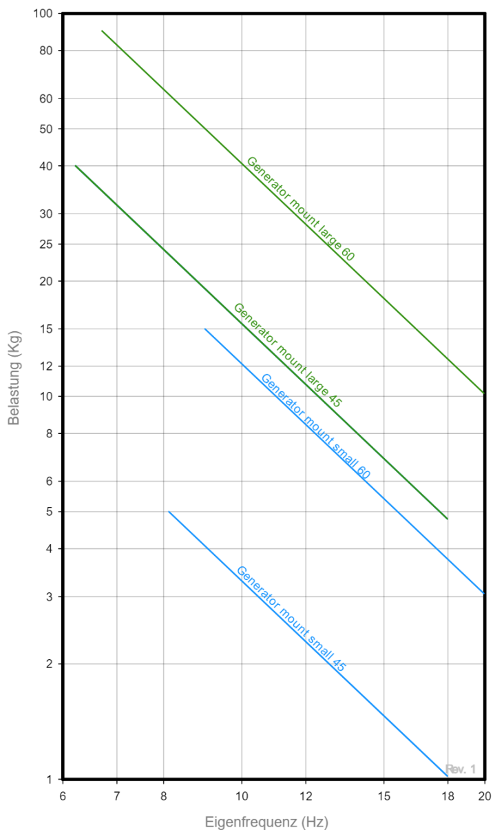
FEDERKENNNLINIE AMC MECANOCAUCHO® GENERATORLAGER V
