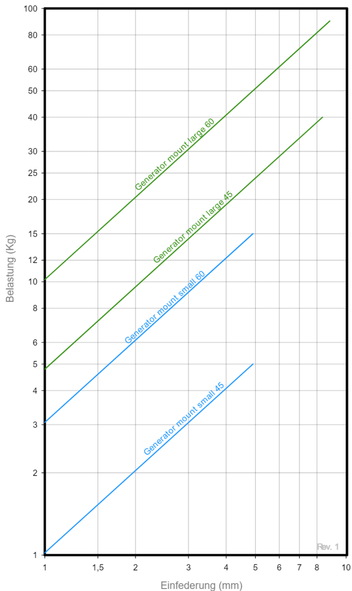
EIGENFREQUENZ AMC MECANOCAUCHO® GENERATORLAGER V
