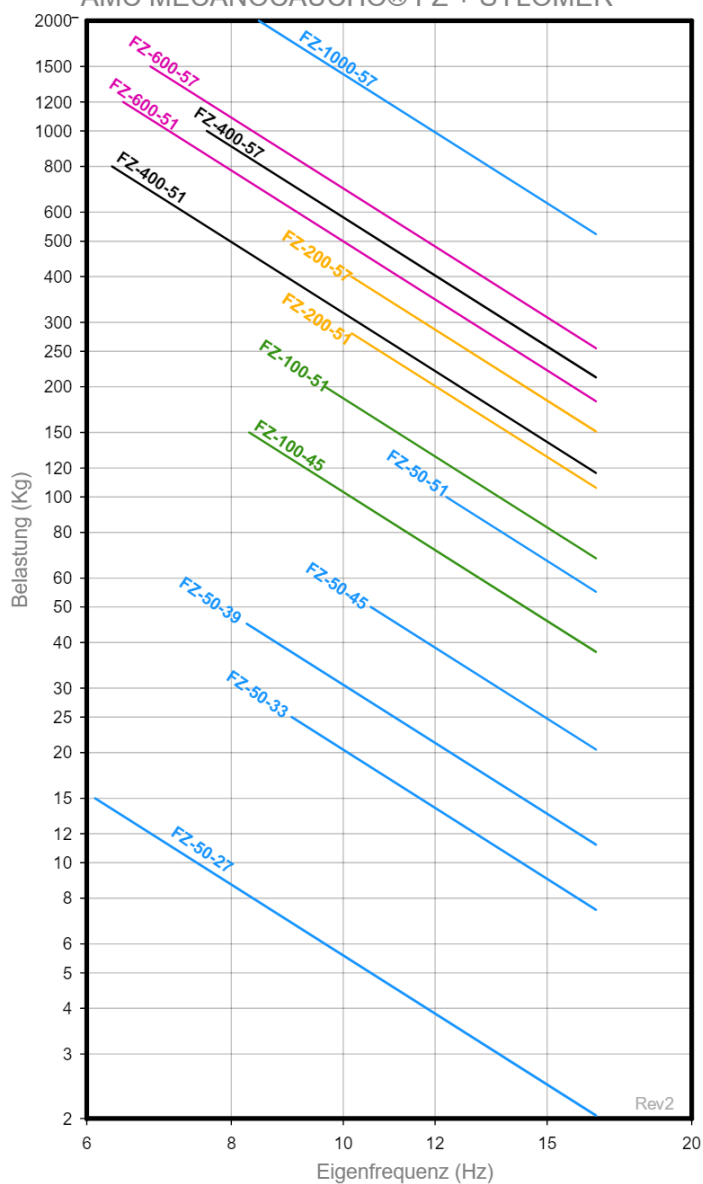
EIGENFREQUENZ AMC MECANOCAUCHO® FZ + SYLOMER
