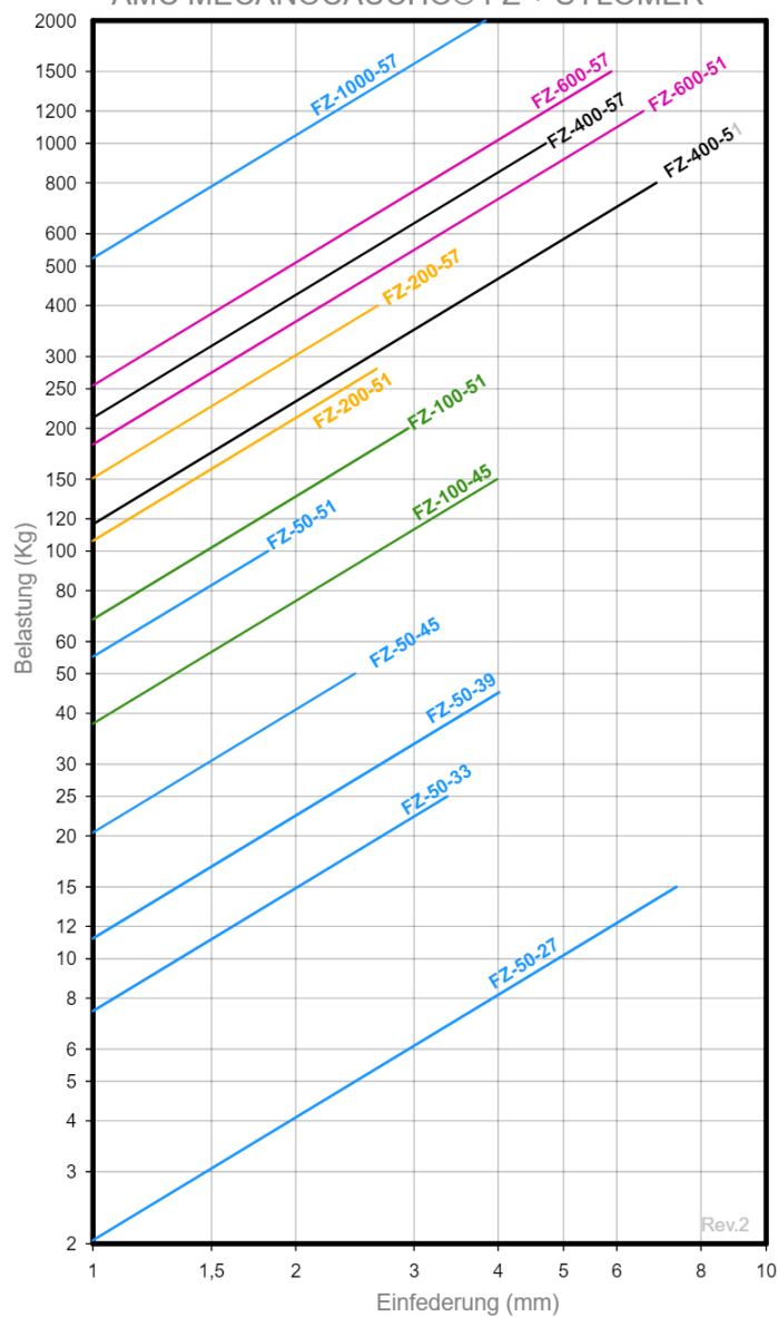
FEDERKENNNLINIE AMC MECANOCAUCHO® FZ + SYLOMER
