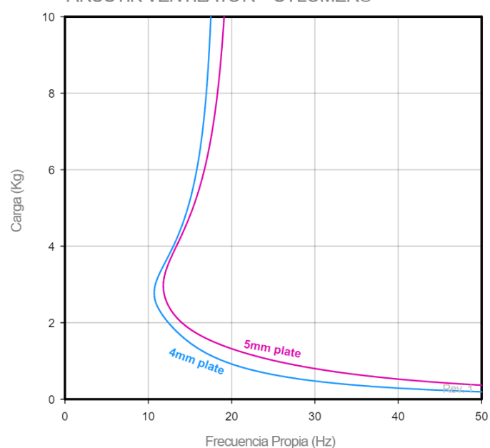
FRECUENCIA PROPIA AKUSTIK VENTILATOR + SYLOMER®
