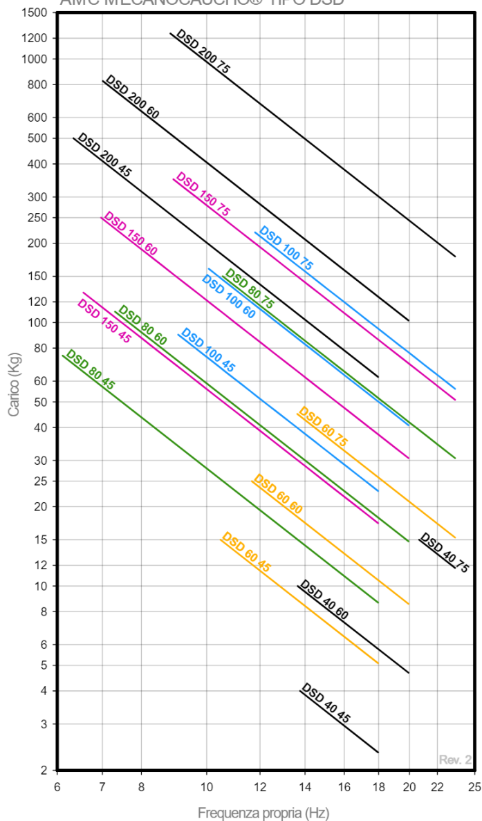
FREQUENZA PROPRIA AMC MECANOCAUCHO® TIPO DSD
