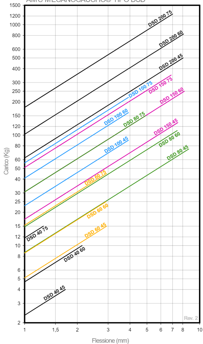
CURVE CARICO FLESSIONE AMC MECANOCAUCHO® TIPO DSD
