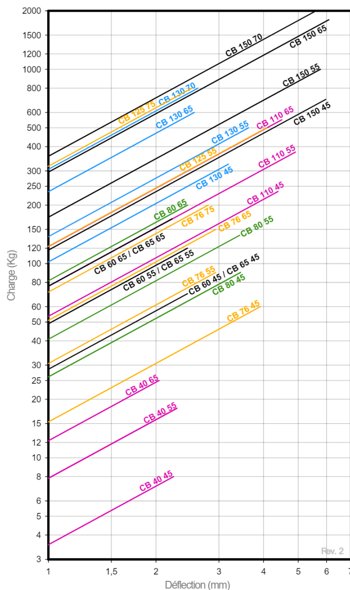
COURBE DE CHARGE FLÉCHE AMC MECANOCAUCHO® SUPPORT ANTIVIBRATOIRE CB
