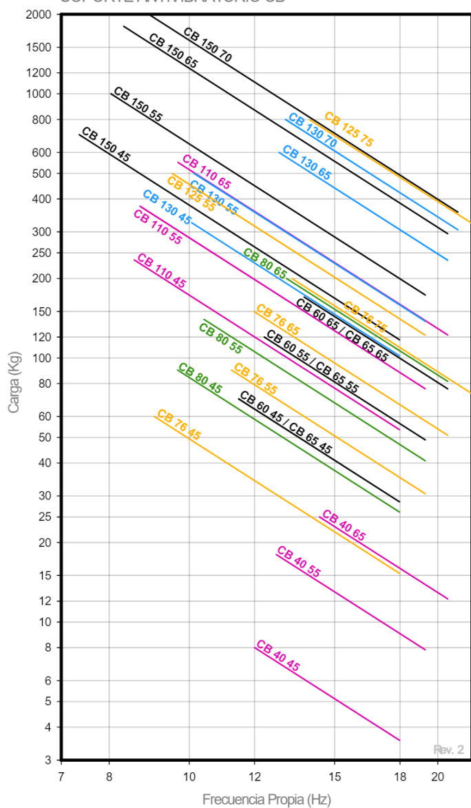
FRECUENCIA PROPIA AMC MECANOCAUCHO® SOPORTE ANTIVIBRATORIO CB
