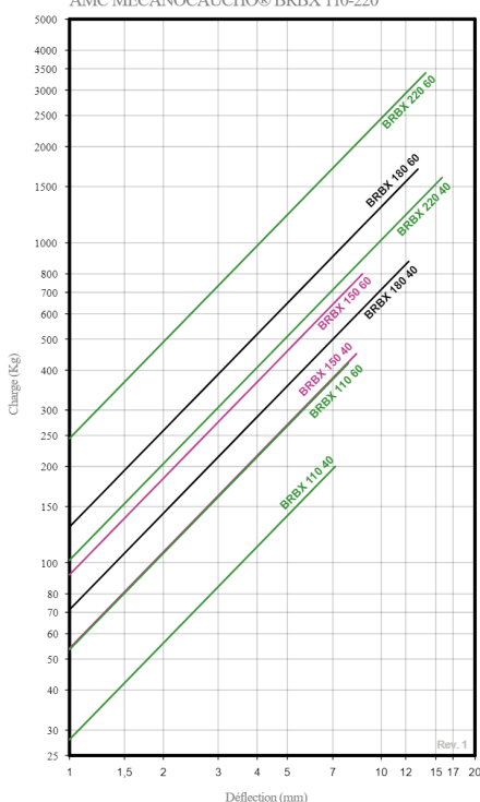
COURBE DE CHARGE FLÈCHE AMC MECANOCAUCHO® BRBX 110-220
