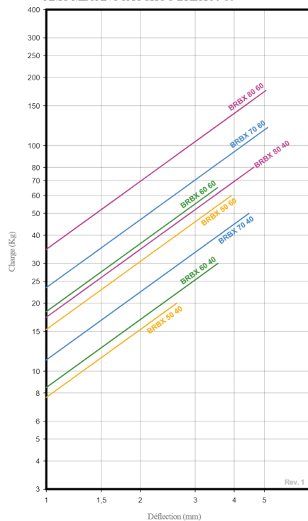
COURBE DE CHARGE FLÈCHE AMC MECANOCAUCHO® BRBX 50-80
