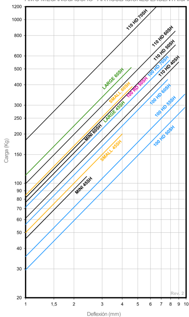
CURVAS DE CARGA FLECHA AMC MECANOCAUCHO® ARTICULACIONES EXCÉNTRICAS
