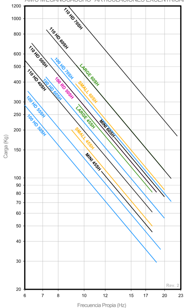
FRECUENCIA PROPIA AMC MECANOCAUCHO® ARTICULACIONES EXCÉNTRICAS
