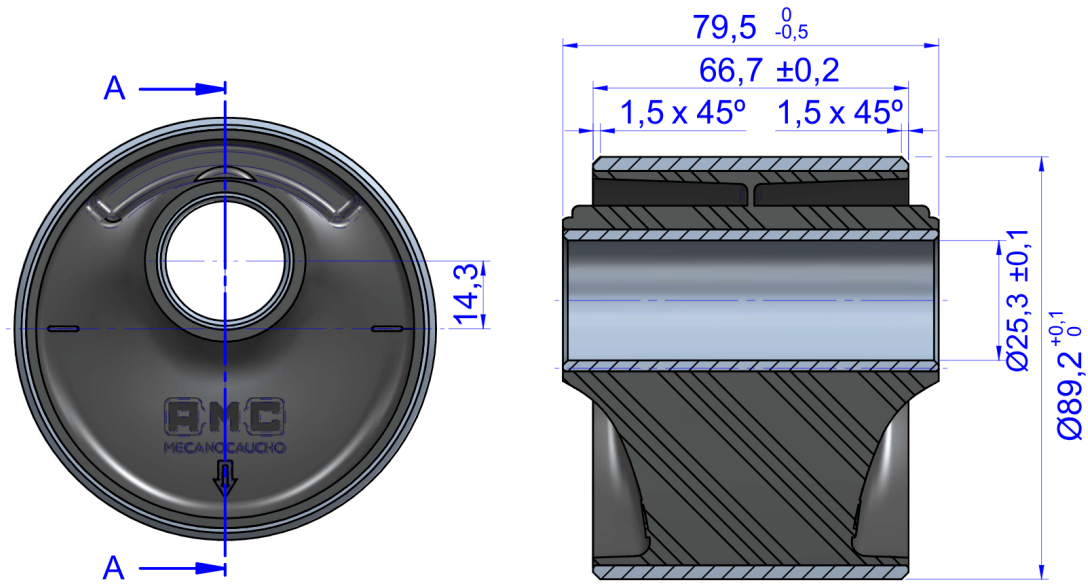
SECTION A-A
