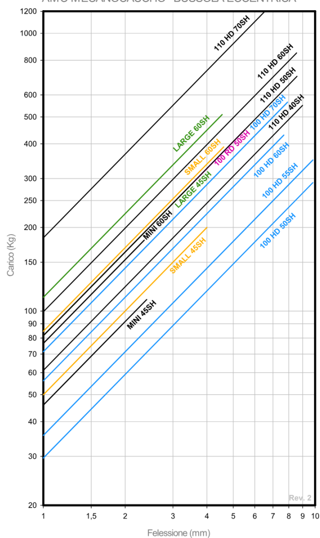
CURVE CARICO FLESSIONE AMC MECANOCAUCHO® BUSSOLA ECCENTRICA
