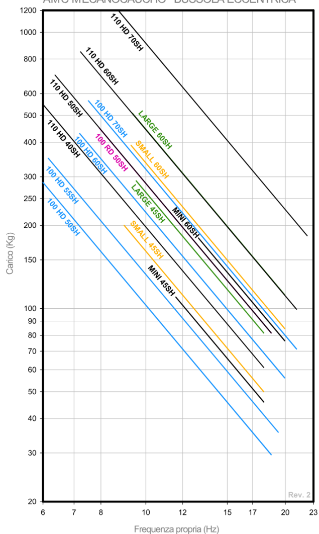
FREQUENZA PROPRIA AMC MECANOCAUCHO® BUSSOLA ECCENTRICA
