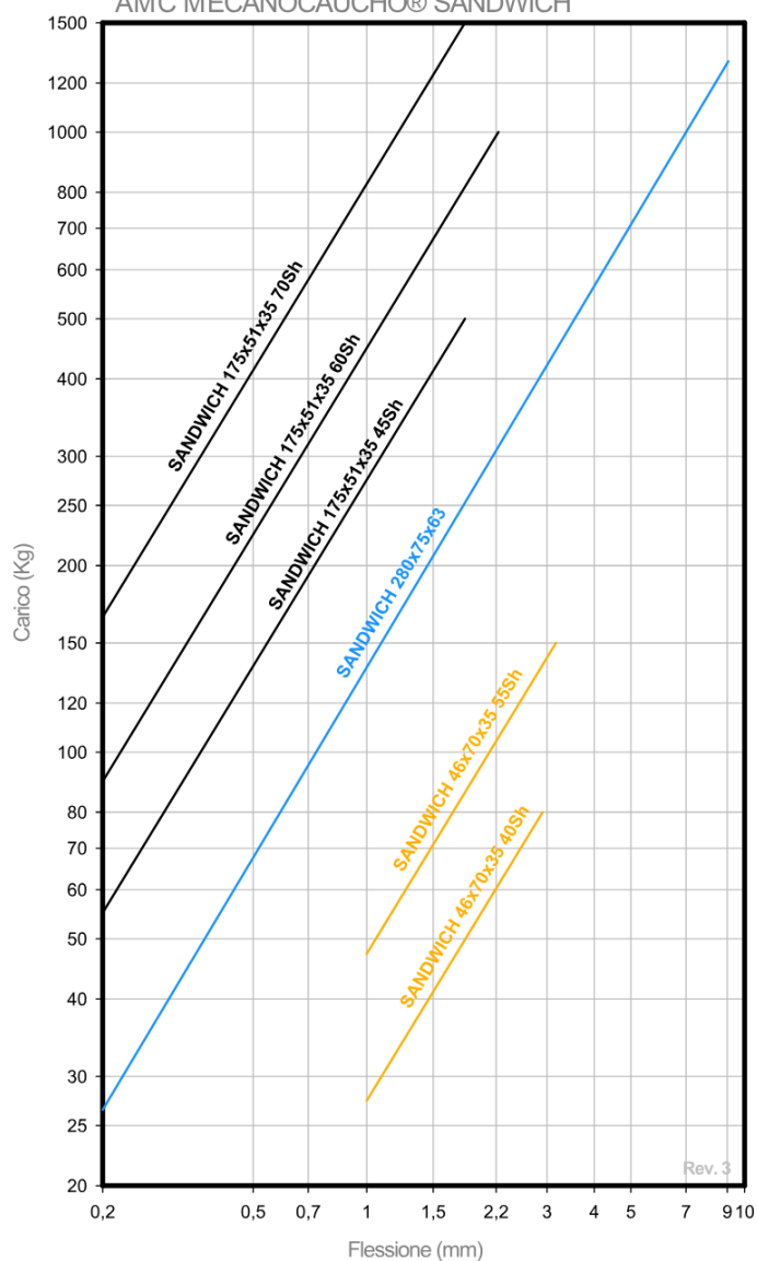
CURVE CARICO FLESSIONE AMC MECANOCAUCHO® SANDWICH
