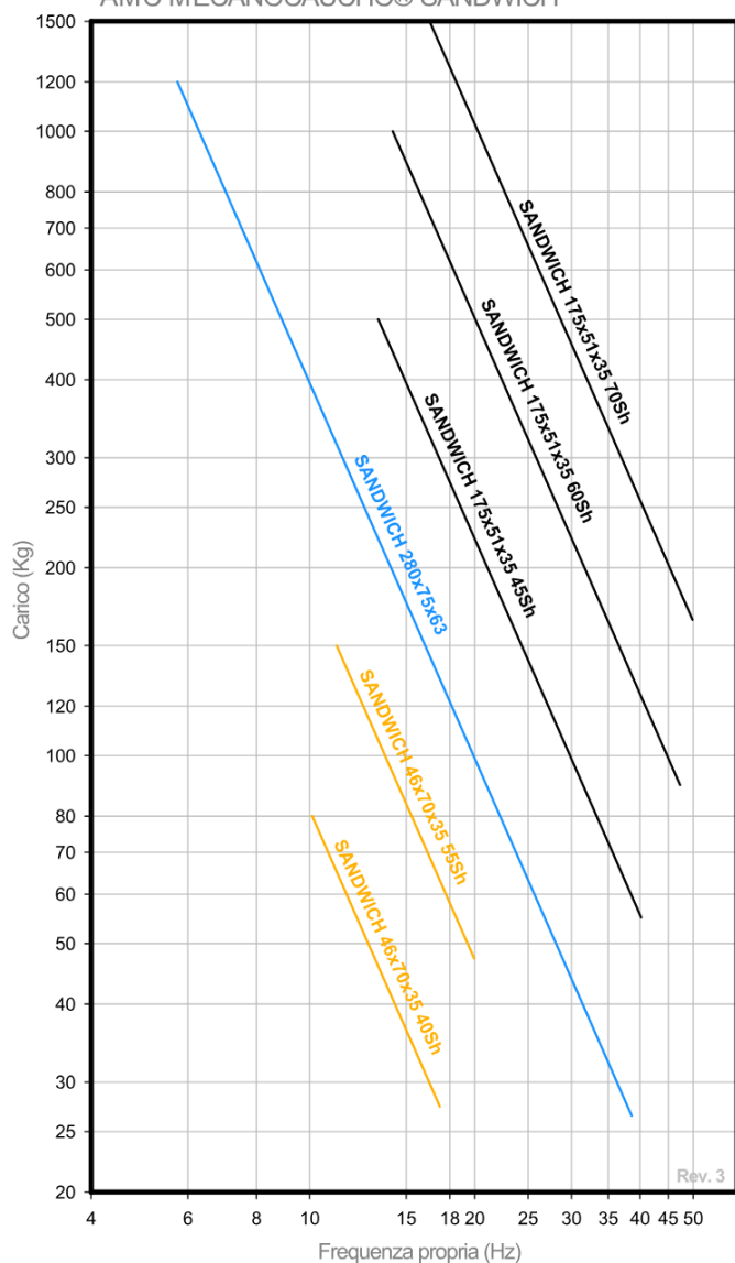
FREQUENZA PROPRIA AMC MECANOCAUCHO® SANDWICH
