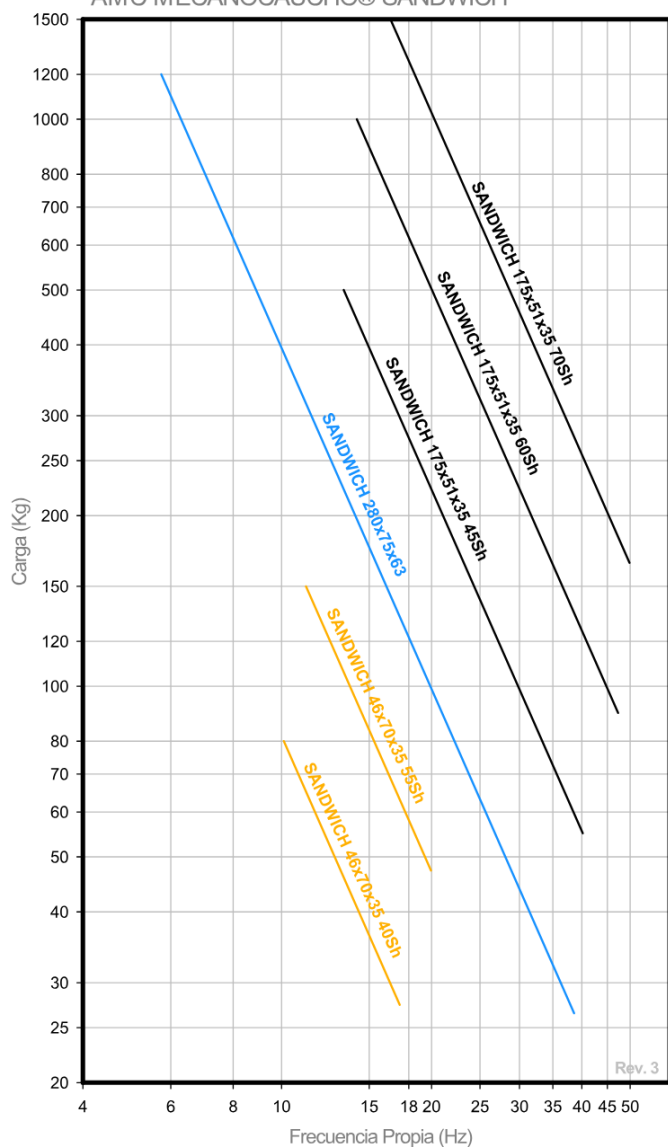
FRECUENCIA PROPIA AMC MECANOCAUCHO® SANDWICH
