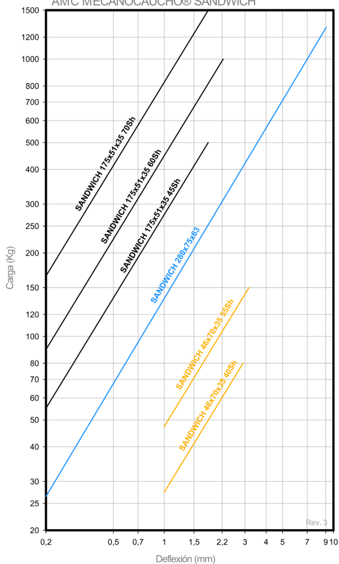
CURVAS DE CARGA FLECHA AMC MECANOCAUCHO® SANDWICH
