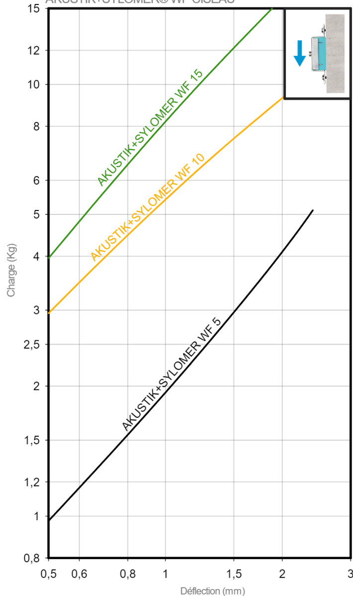
COURBE DE CHARGE FLÈCHE AKUSTIK+SYLOMER® WF CISEAU
