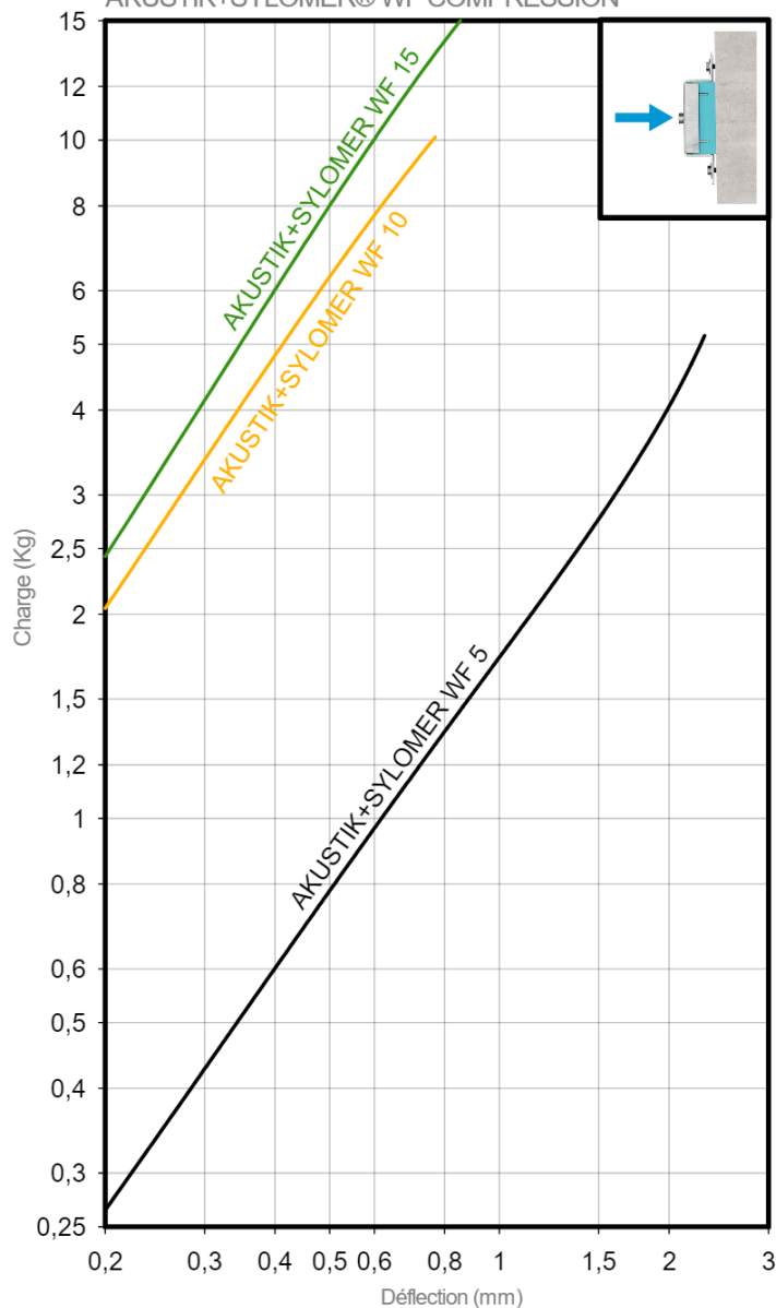
COURBE DE CHARGE FLÈCHE AKUSTIK+SYLOMER® WF COMPRESSION
